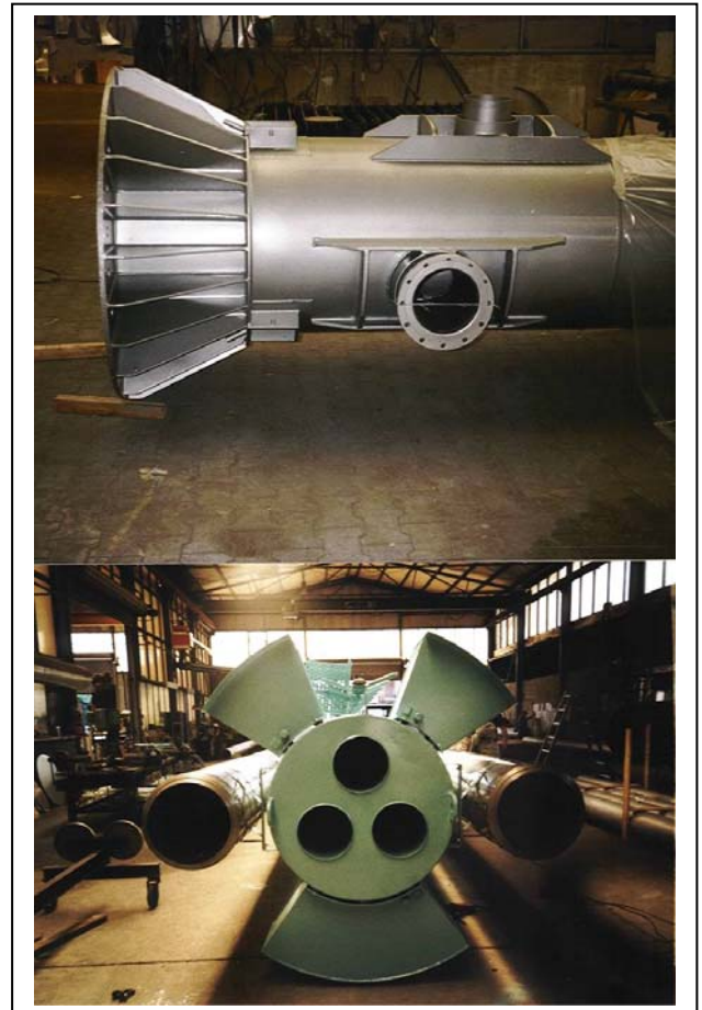
Dreizügige Anlage oben - Anschlußsituation Kom.: BHKW-Anlagen Höhe: 12 m Züge: 2x 250 mm, 1x 100 mm Tragmantel: 900 mm Typ: Triomat-S3E-L
